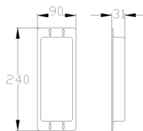
Antenna
